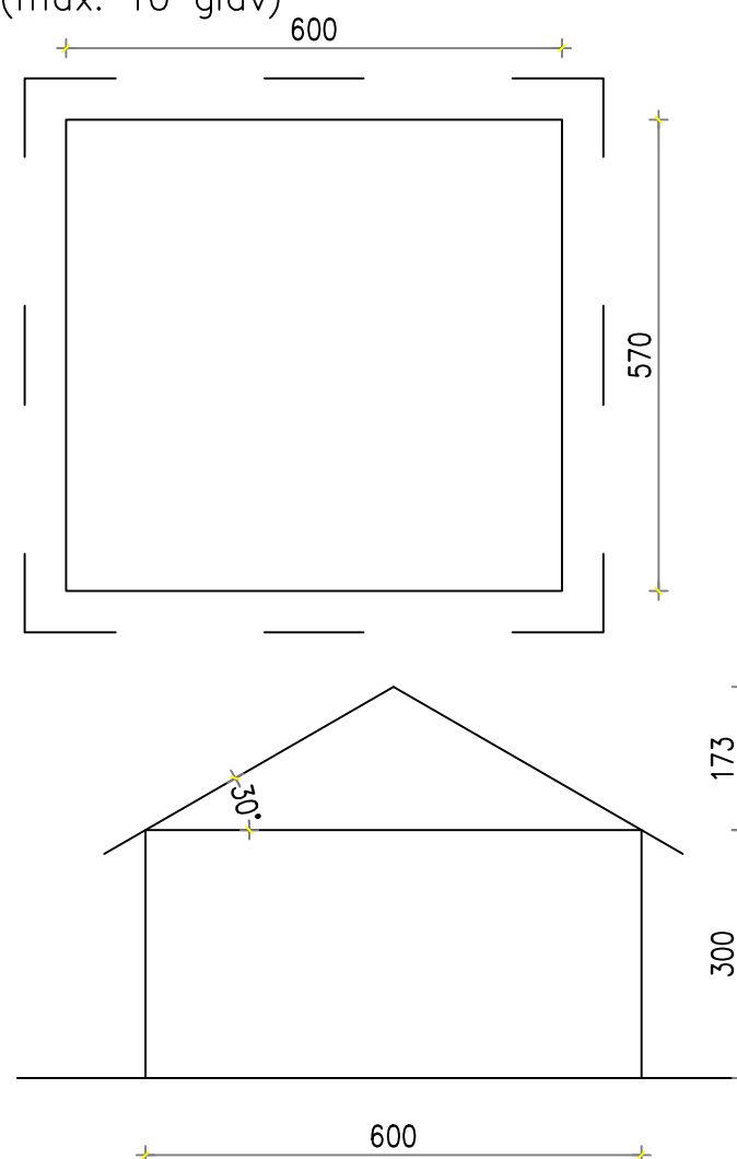
HLEV ZA GOVEDO (tip A) (max. 10 glav)
