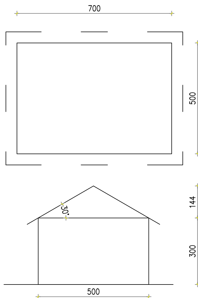
SUŠILNICA MESA (tip B)
